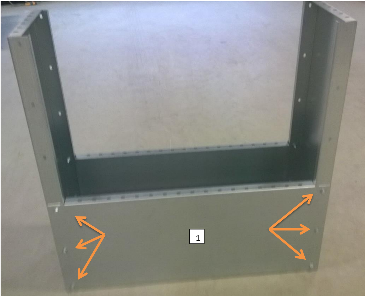
1. Kokoa jalusta ylösalaisin käännettynä tasaisella alustalla.
