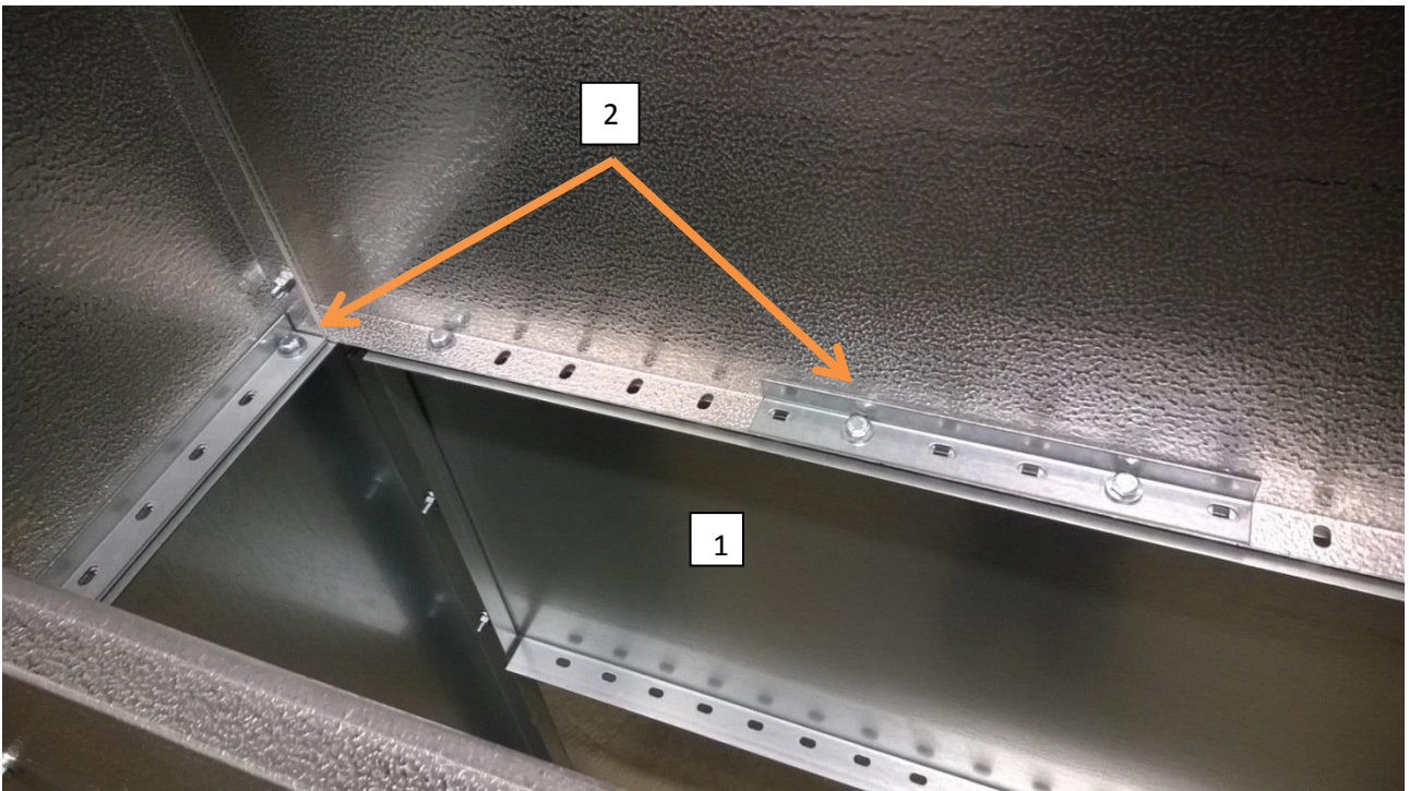
2. Kaappi ja jalusta kiinnitetään toisiinsa pulteilla ja tukiraudoilla. Tukiraudat asetetaan alumiinikaapin sisäpuolelle.
